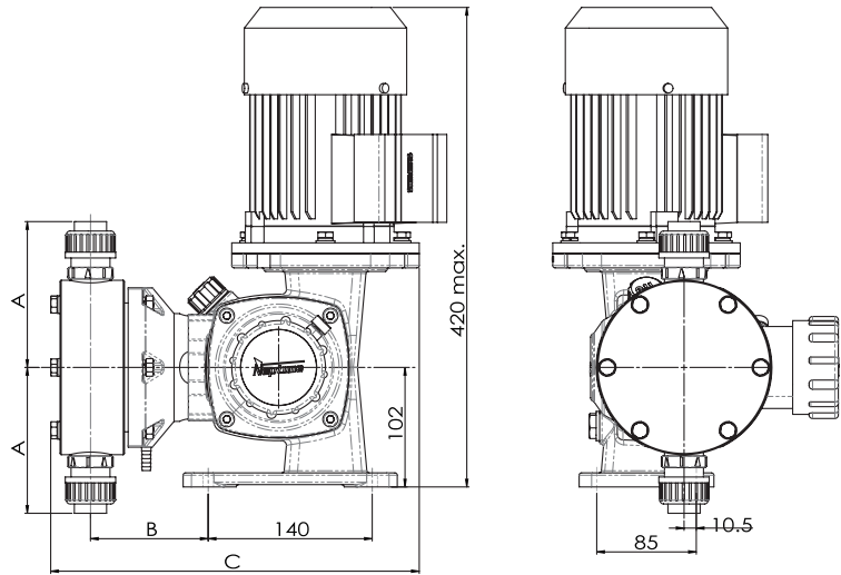
NPBG 外形及尺寸
