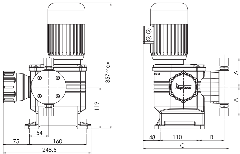
NPBG 外形及尺寸
