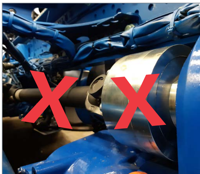
无 需传动轴 无 力矩限制器
