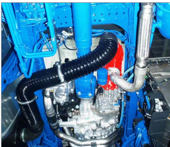
将压缩机组件直接安装在 齿轮箱上
