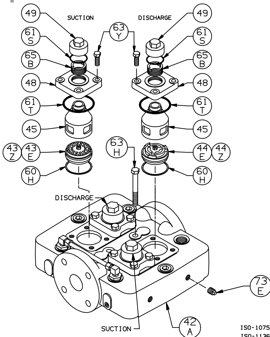
Head Assembly: HDL642C|B, HDL643C|B
