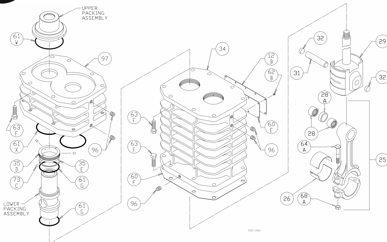
Crosshead Assembly: HD603C, HDL603C, HDL643C
