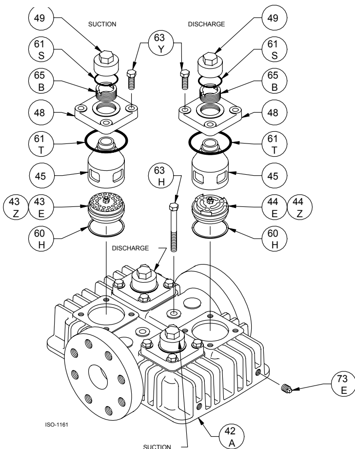
Head Assembly: HD601B|A, HD602C|B|A, HD603C|B|A
