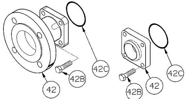
ANSI FLANGE
